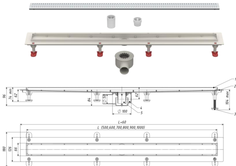
Рис. 1 – Габаритные размеры
